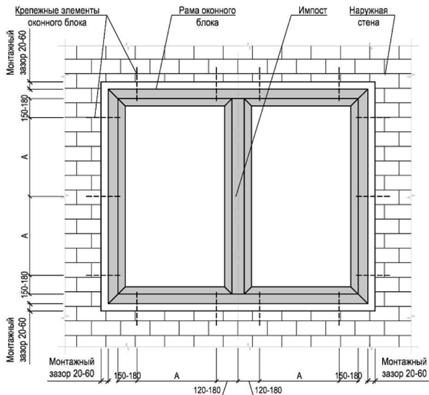
Схема закрепления оконного блока в светопроеме
