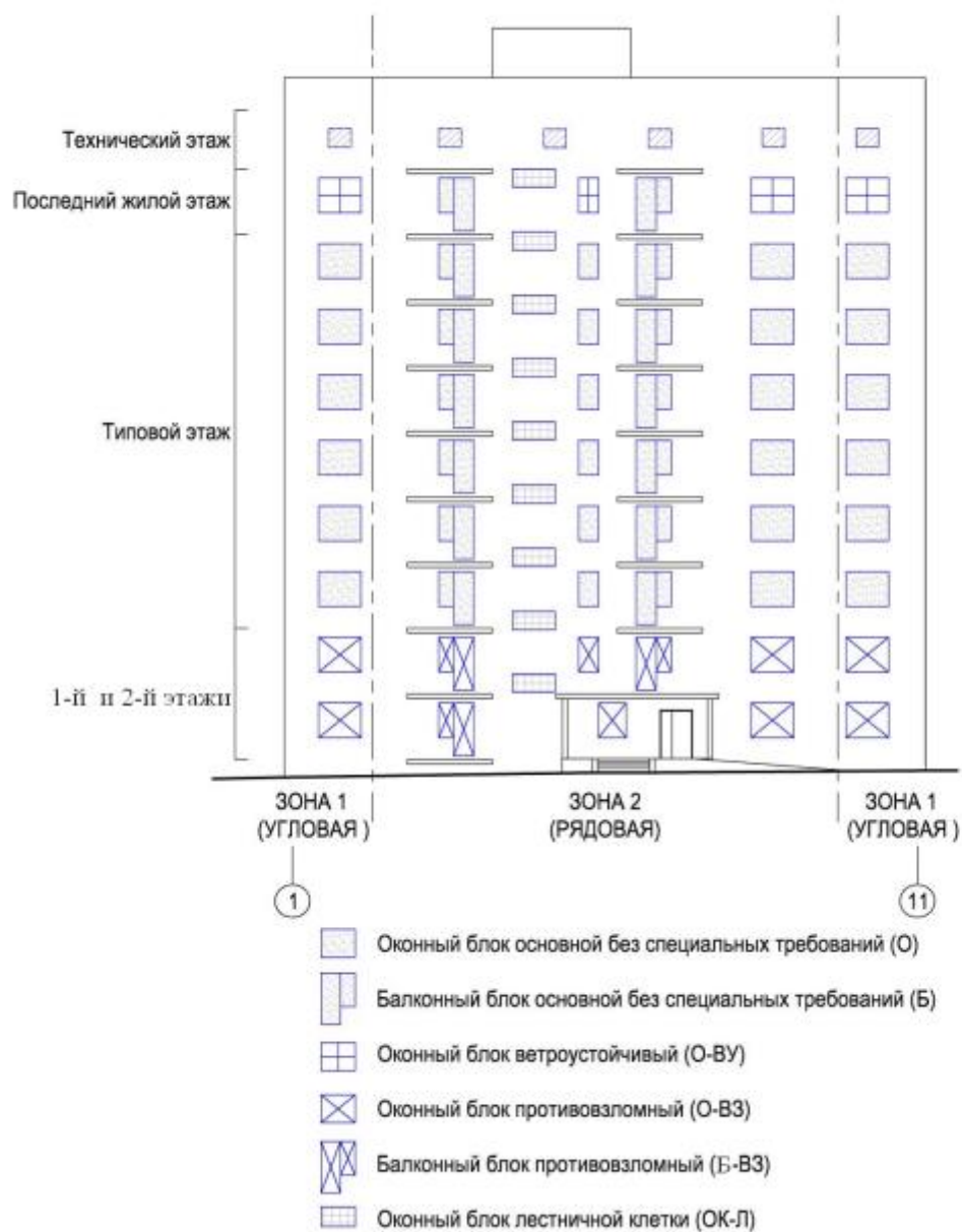
Рисунок Г.1 – Пример функционального зонирования фасада здания по требованиям к оконным блокам
