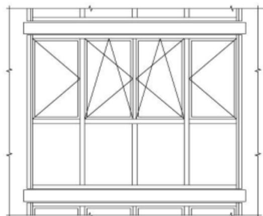
Рисунок Д.2 – Примеры конструкций наружного остекления
