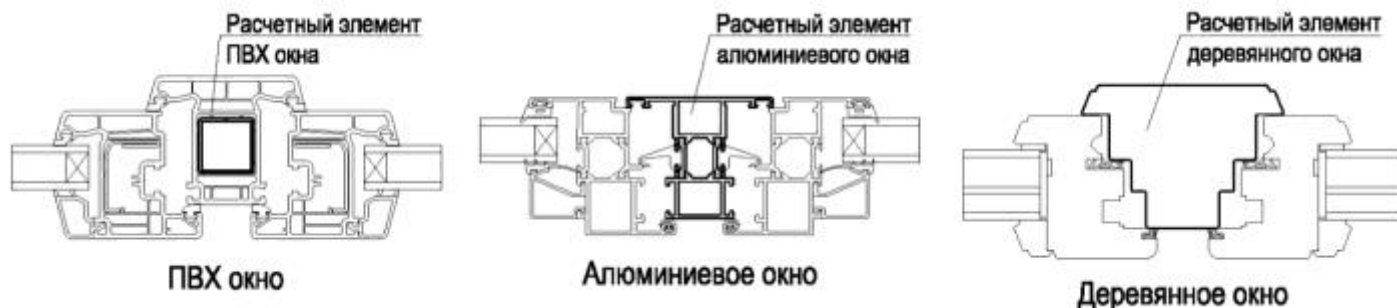
Рисунок Б.5 – Расчетные элементы (вертикальные импосты) окон различной конструкции
