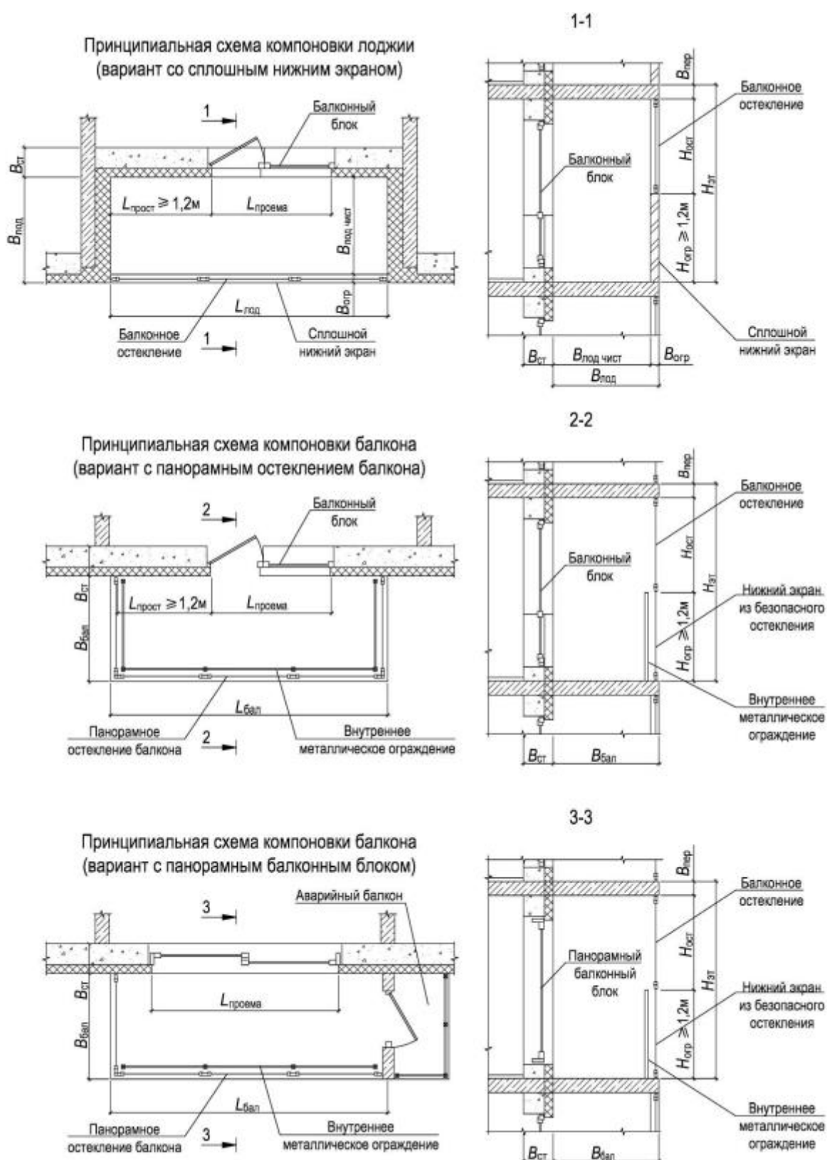
Рисунок Д.1 – Основные варианты архитектурно-планировочные и конструктивных решений остекленных балконов и лоджий
