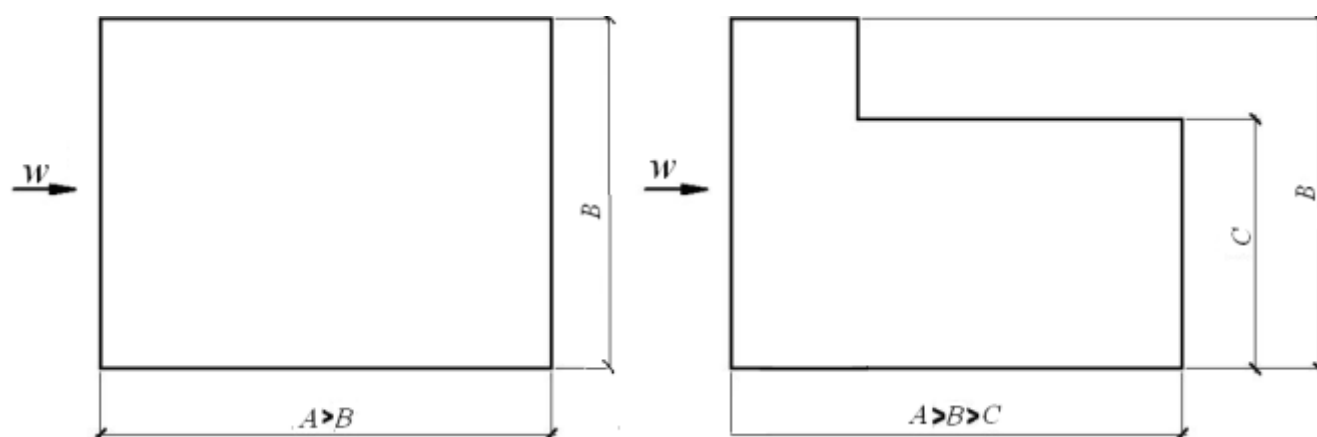
Рисунок Б.1 – Схема определения расчетного направления ветра
